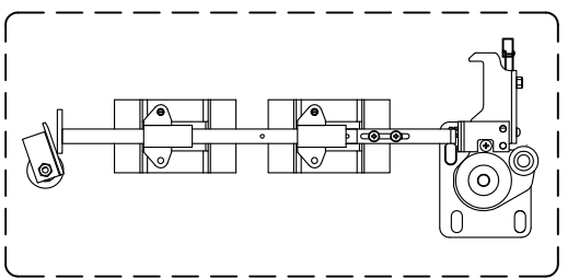
当OPH=2300~2400 时开锁装置按下图
