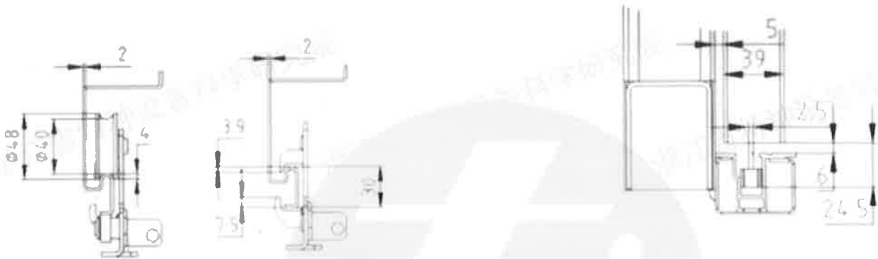
图1 上部导向和保持装置侧视图
